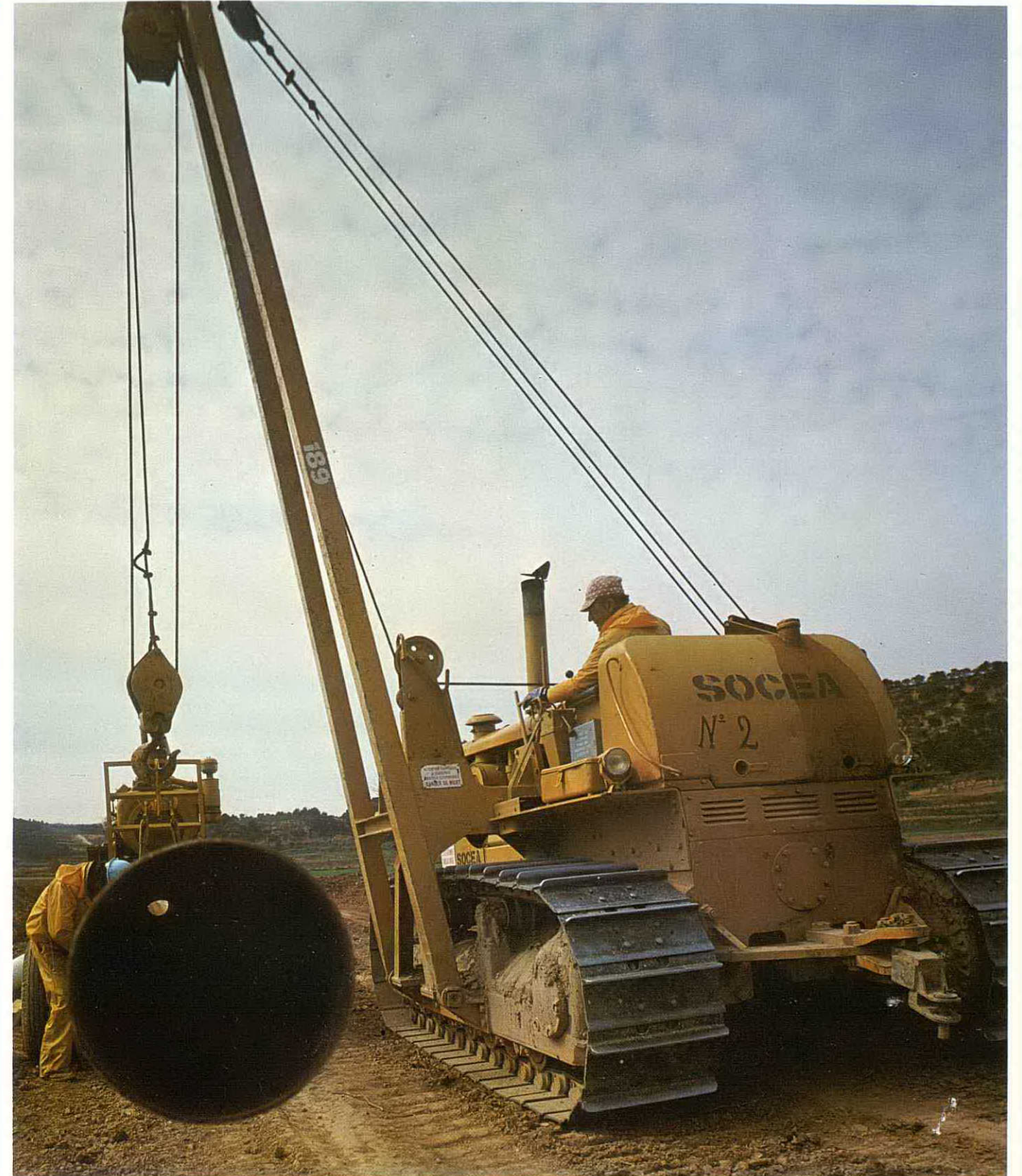
Montaje del oleoducto Tarragona-Zaragoza
