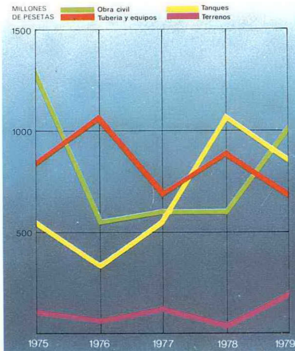
DESGLOSE DE LAS INVERSIONES EN INSTALACIONES DE ALMACENAMIENTO Y EDIFICIOS
